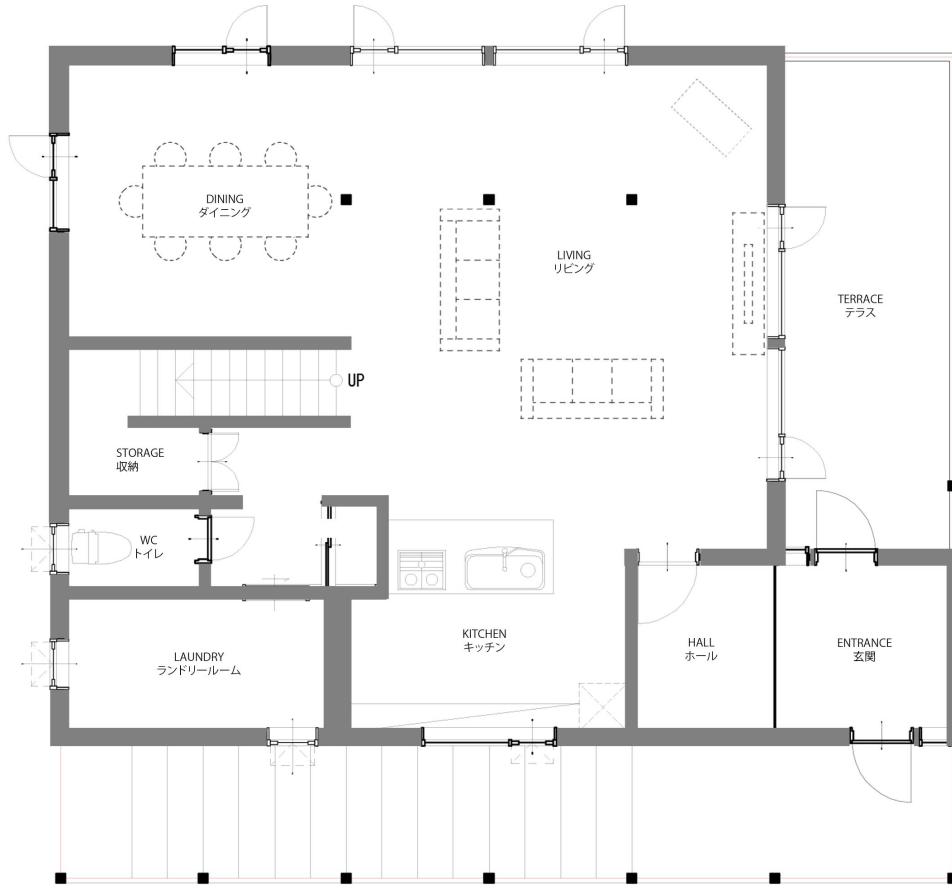
1階平面図 First Floor
