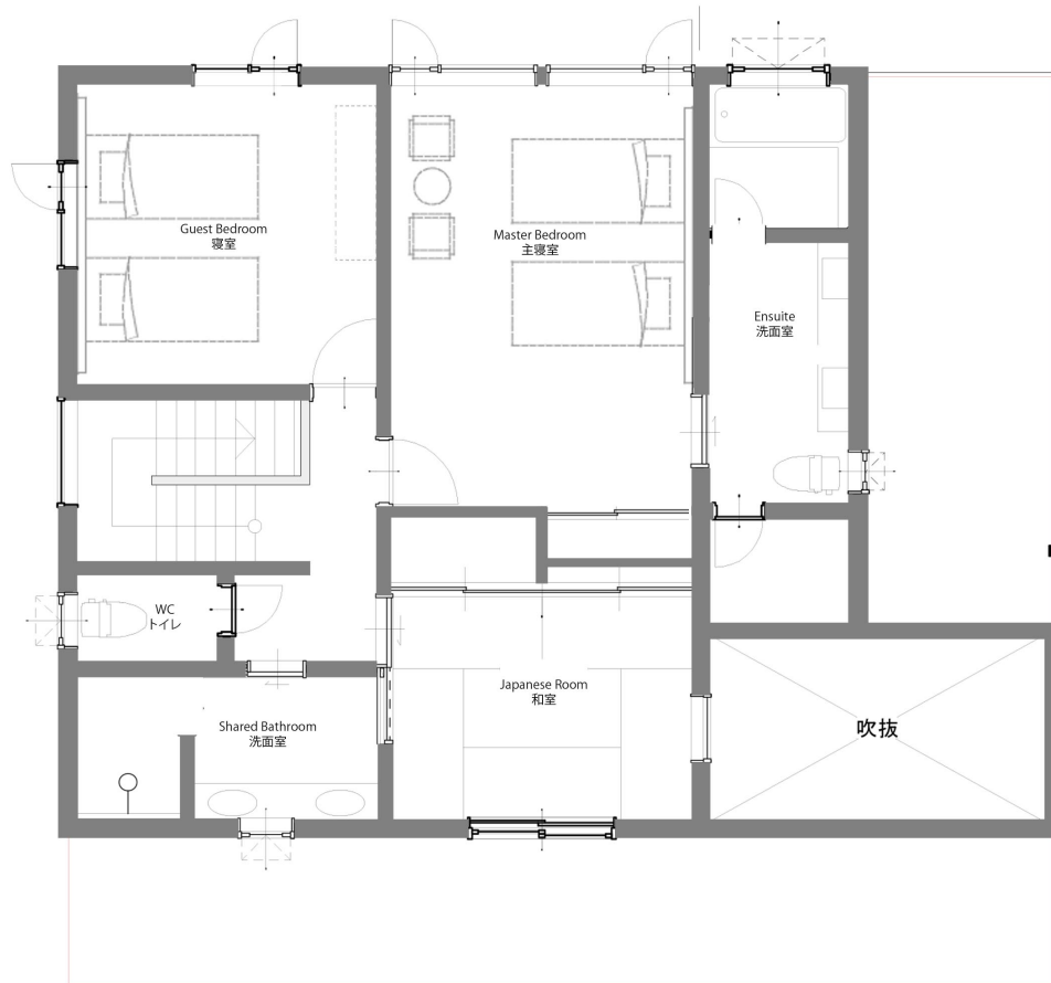
2階平面図 Second Floor
